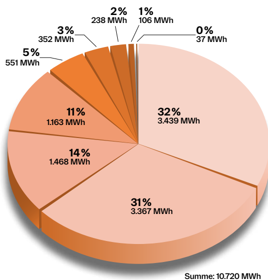
Starlinger Energieverbrauch 2023/24 in MWh Aufteilung in %
